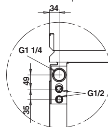
Dettaglio E
